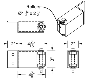
01 Guide Roller Scale: NTS
